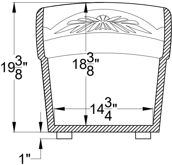
SECTION A-A1
