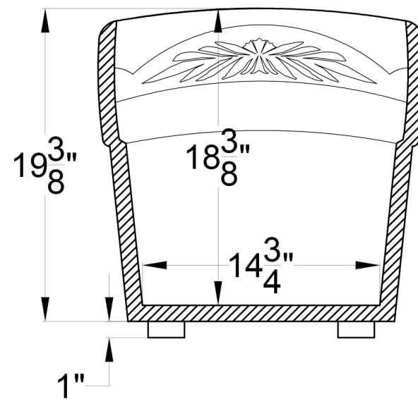
SECTION A-A1
