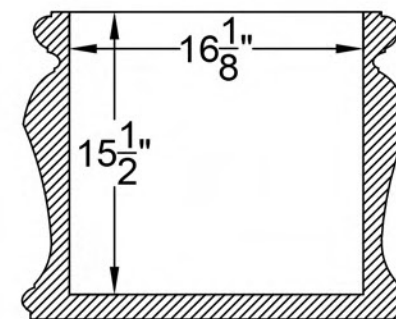
SECTION A-A1
