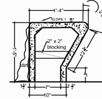
SECTION A-A1
