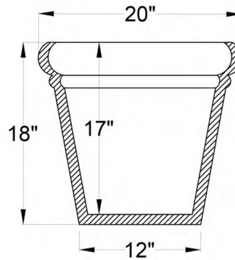
SECTION A-A1
