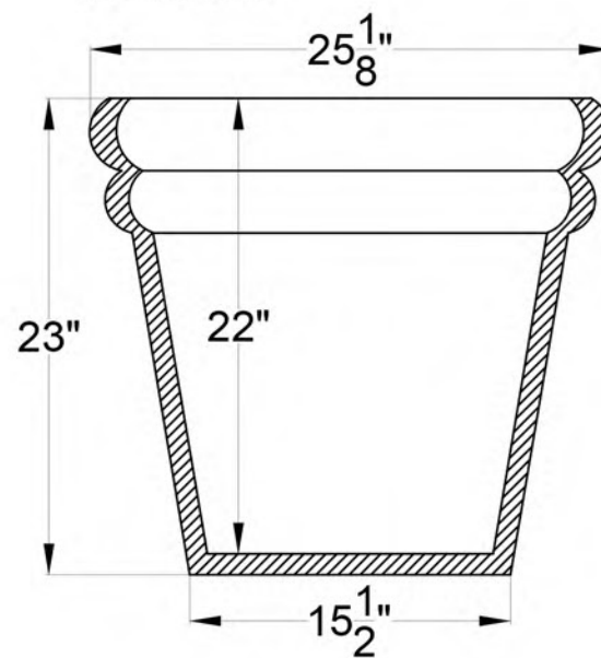
SECTION A-A1
