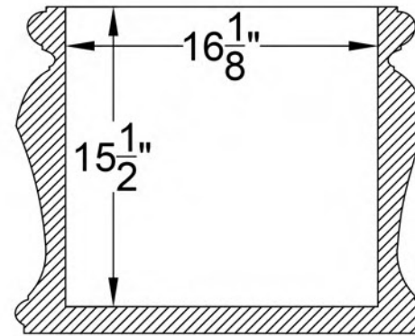
SECTION A-A1
