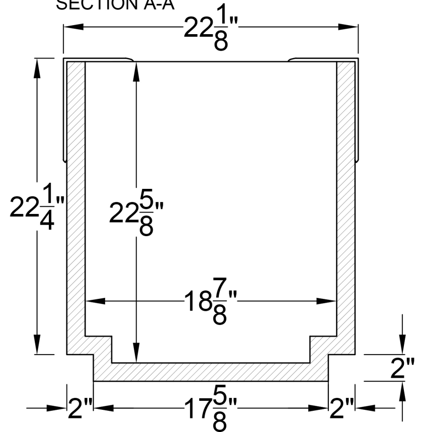
SECTION A-A
