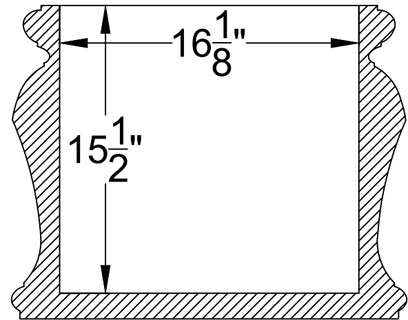
SECTION A-A1
